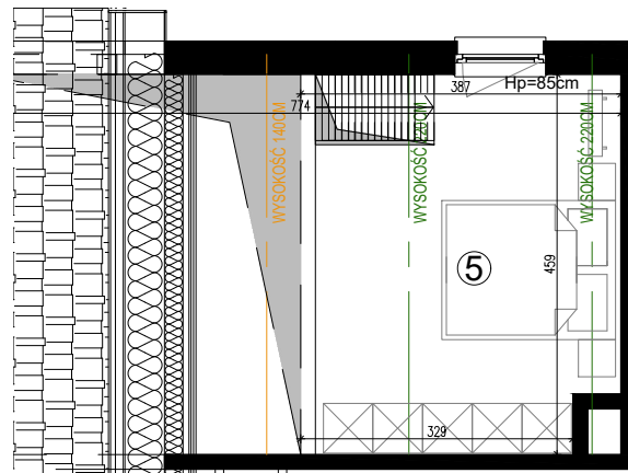
POZIOM ANTRESOLI
