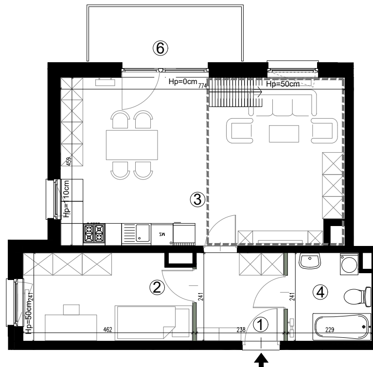
POZIOM KONDYGNACJI +3
