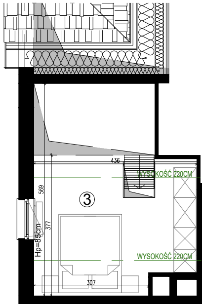
POZIOM ANTRESOLI
